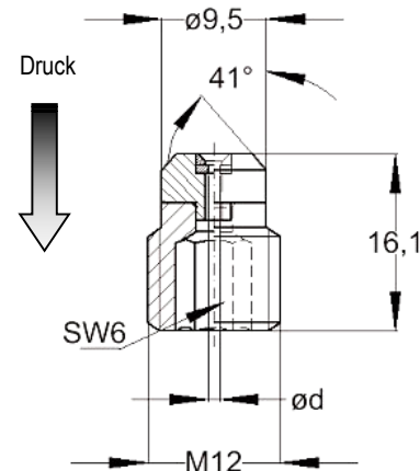
Saphir Einschraubdüse 018S-M12
