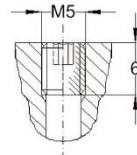
Kunststoff Blinddüse / Stopfen 056P eingeklebt
