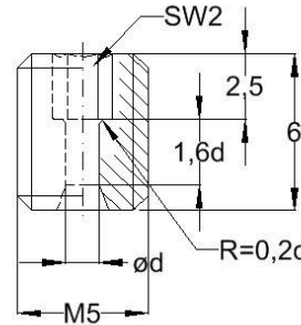
Kunststoff - Drosselschraube Gewindedüse M5x6 Typ 056 P-ø1,00 mm
