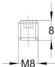
Verschlussstopfen, Blindedüse TN 6212.5000.1
