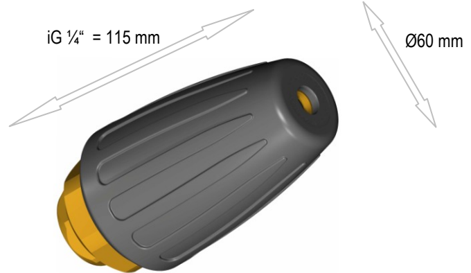
MonoWhirl 500-MS
